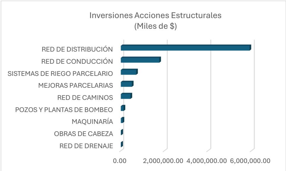
Grafica 3.1. Acciones estructurales e inversión total considerada en el plan director del Distrito de Riego 100.
